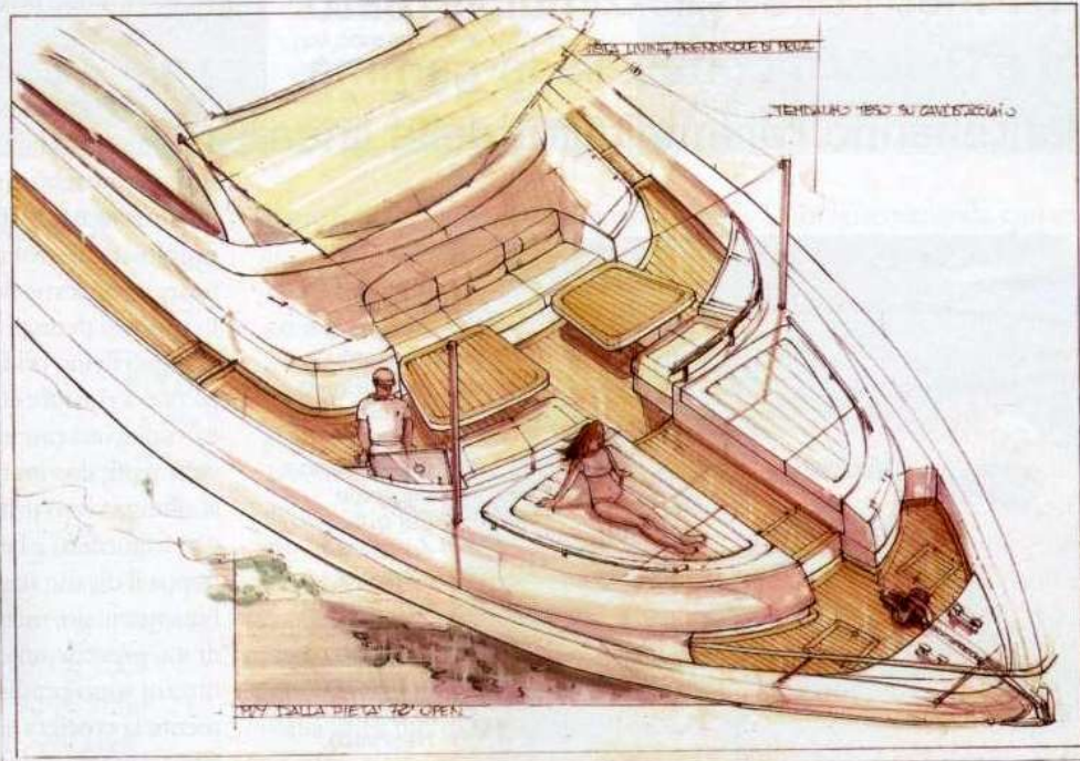
A sinistra, la zona del ponte di prua è quella che più caratterizza questa nuova ammiraglia del cantiere Dalla Pietà. Il tradizionale prendisole è stato sostituito da un vero e proprio pozzetto attrezzato con divani, tavoli, prendisole e una stazione di comando, una soluzione veramente innovativa.
